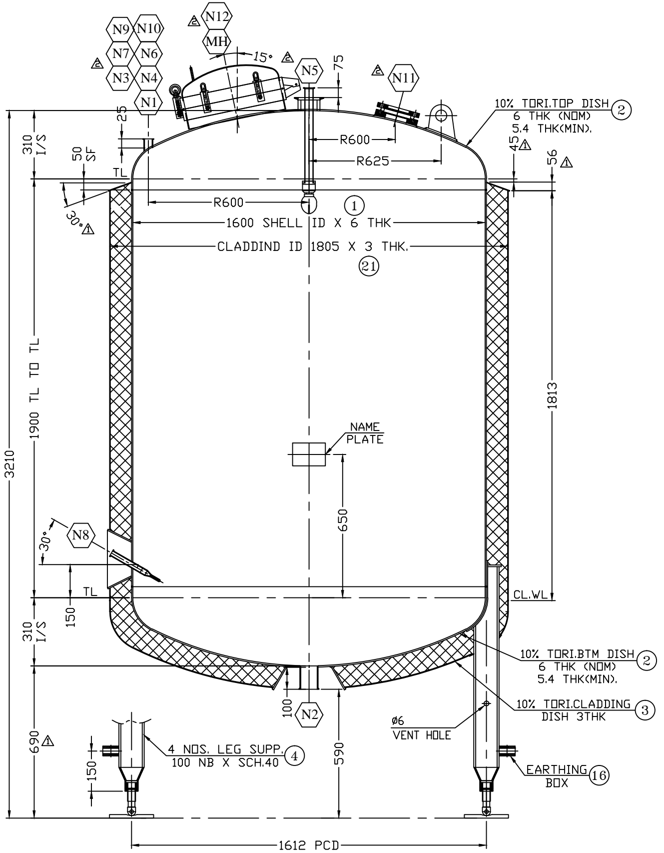
△ ELEVATION
